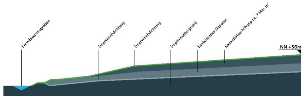
Abb. 3: Schematische Darstellung der Kapazitätserhöhung
